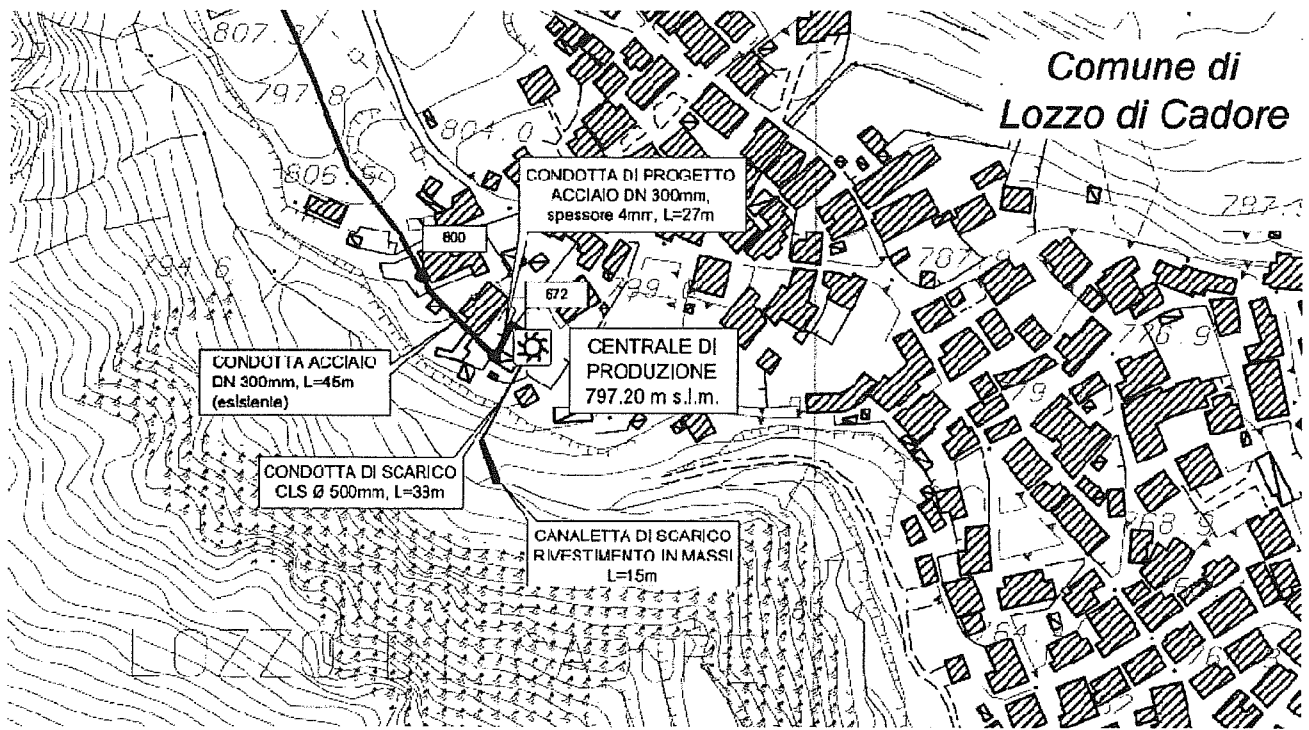
Estratto C.T.R. e PLANIMETRIA CATASTALE con indicazione CONDOTTA DI SCARICO
